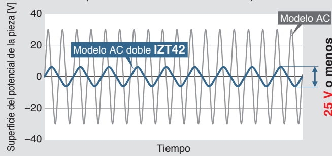
Comparación de la amplitud de potencial entre el modelo AC y el modelo AC doble (Altura de instalación del sensor: 300 mm)
