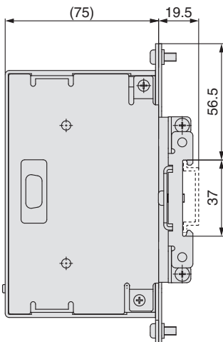
Quando se usa fijación de montaje sobre raíl DIN (IZT40-B1)
