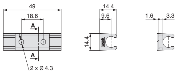
Vista transversal A-A
