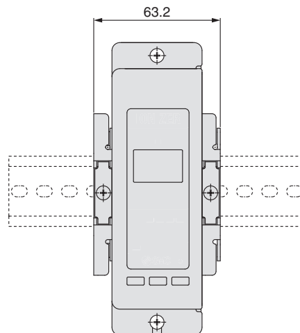
Quando se usa fijación de montaje sobre raíl DIN (IZT40-B1)
