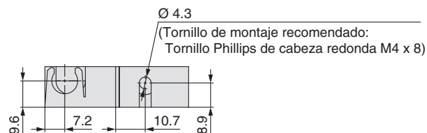
Vista transversal A-A
