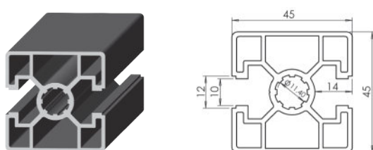
Perfil 45x45 2S 180º Profile 45x45 2S 180º
