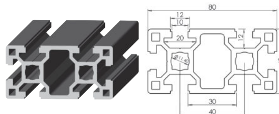
Perfil pesado 40x80 Heavy profile 40x80
