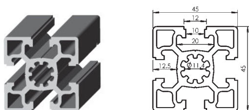
Perfil pesado 45x45 Heavy profile 45x45
