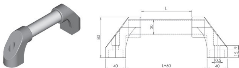
SUJECIÓN ASA TUBULAR / HOLDER
