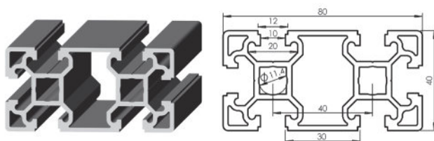
Perfil estándar 40x80 Standard profile 40x80
