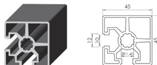
Perfil 45x45 2S 90º Profile 45x45 2S 90º
