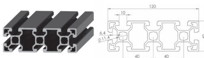
Perfil estándar 40x120 Standard profile 40x120
