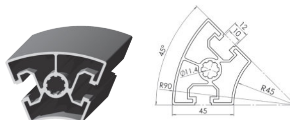
Perfil 45x45° Profile 45x45°
