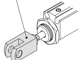
Montaje de la horquilla hembra
