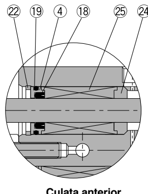
Culata anterior
