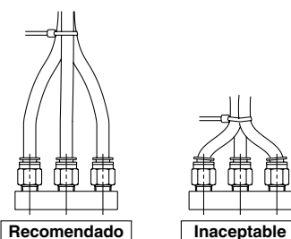
Fig. 2 Doblado de los tubos por medio de bandas
