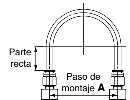
Fig. 1 Configuración de conexión recomendada
